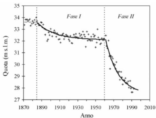
Figg. 1 e 2. A sinistra il trend temporale della quota del fondo dell'alveo a Cremona con evidenziate le fasi di abbassamento del fondo (modificato da Lamberti e Schippa, 1994 –by Massimo Rinaldi) 13 . A destra la rappresentazione sintetica delle evidenze di abbassamento del fondo del Po e dei suoi principali affluenti. I dati riportati indicano come gran parte, circa il 40% dei corsi d'acqua, sia interessata da fenomeni medi e significativi di abbassamento (fonte: AdbPo "Caratteristiche del bacino del fiume Po e primo esame dell'impatto ambientale delle attività umane sulle risorse idriche – aprile 2006").
