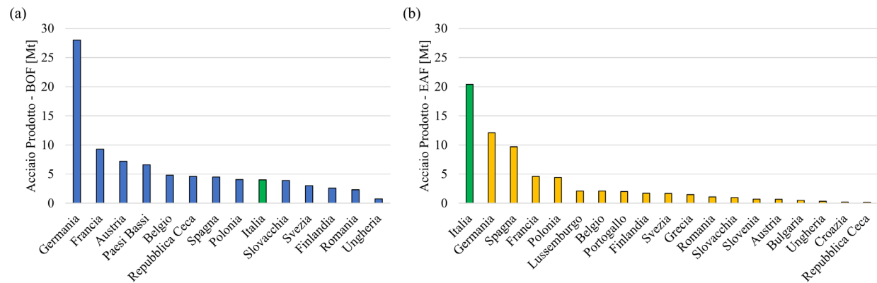
Figura 4 – a) Produzione europea di acciaio primario con tecnologia BF - BOF nel 2022; b) Produzione europea di acciaio da rottame con tecnologia EAF nel 2022
